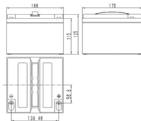
外形尺寸
